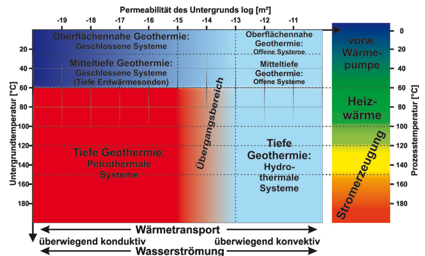
Abb. 3.1.7.2: Definitionsmöglichkeiten für geothermische Nutzsysteeme in Abhängigkeit von der Lagerstätten-Permeabilität und der Erschließungsteufe | Quelle: Sass 2012
