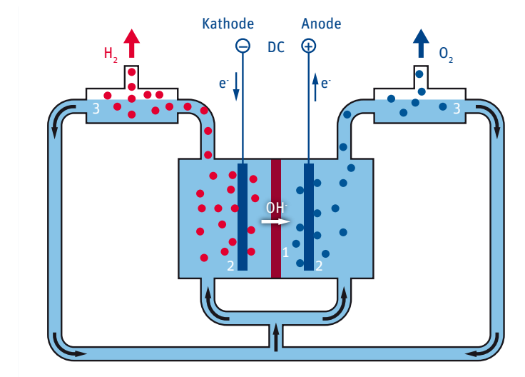
Abb. 3.3.4.1.1: Funktionsprinzip der alkalischen Wasserelektrolyse | Quelle: Dr. U.R. Fischer
